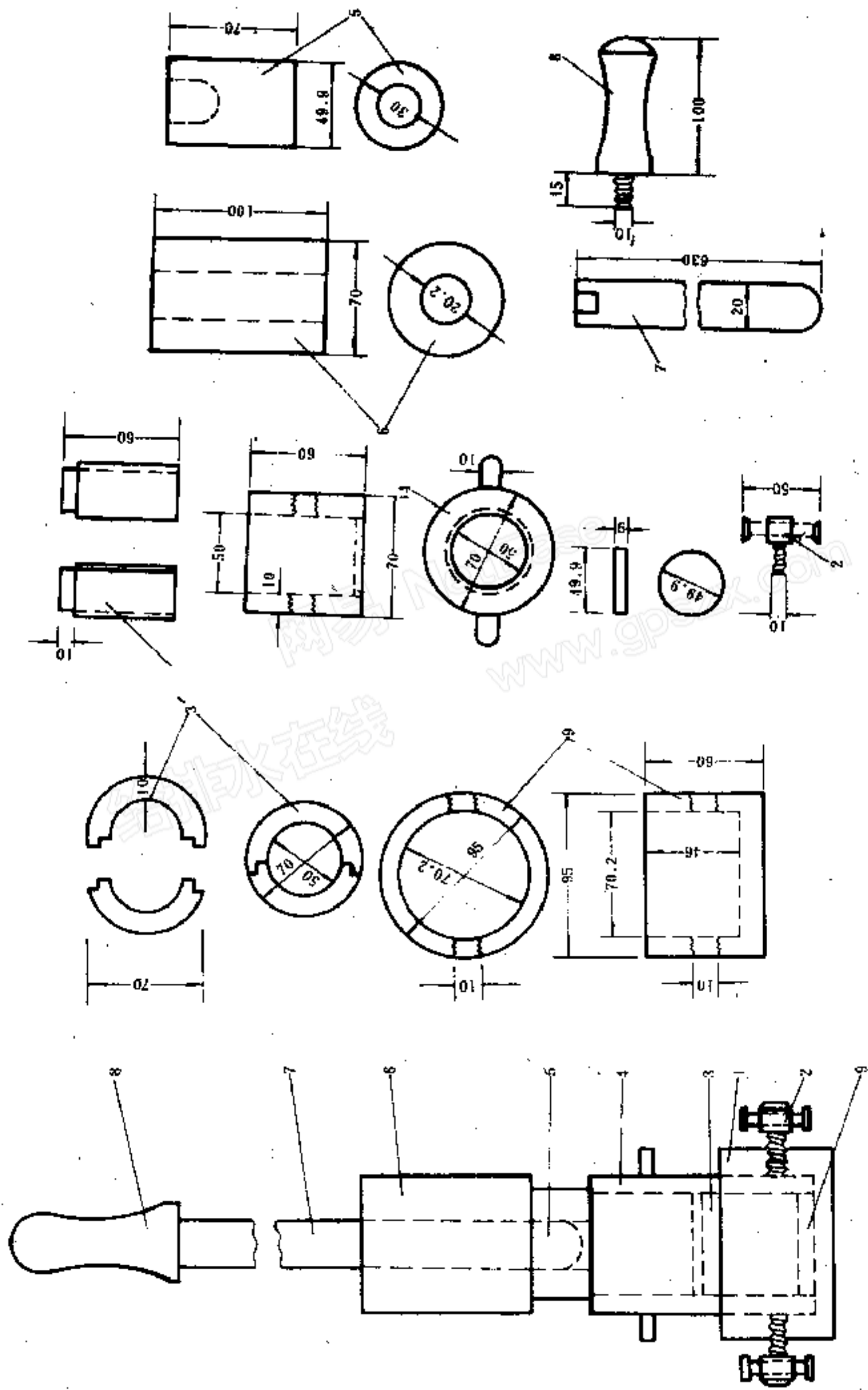
附图 4.2 100cm³ 小型击实仪
