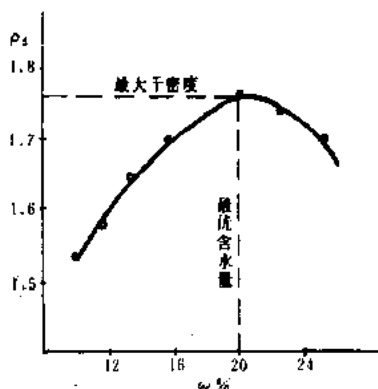
附图 4.1 \rho_d \sim \omega 关系曲线
