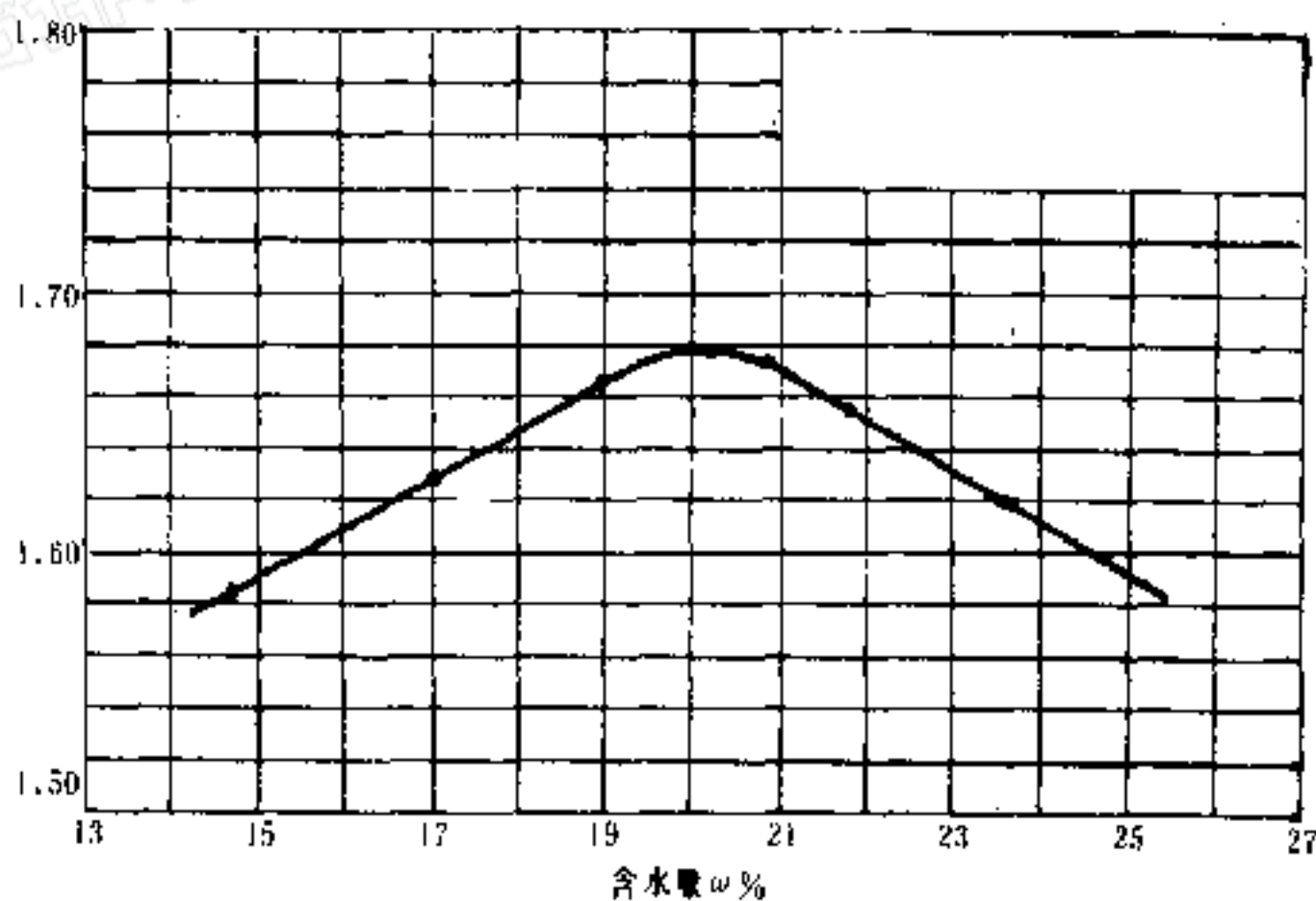
附图 4.3 含水量与干密度关系曲线
