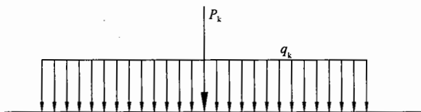
图 10.0.2-1 车道荷载
