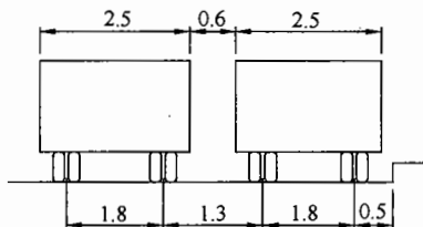
(6) 汽车荷载的横向布置
